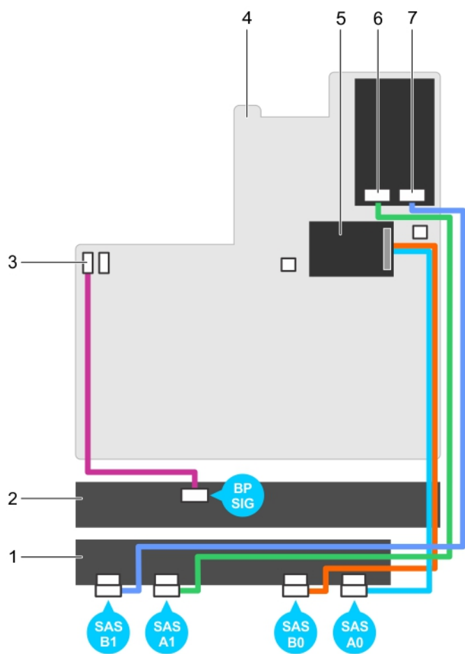
图 55: 布线图 - 2.5 英寸 (x24) SAS/SATA 背板 - (选项 2)
