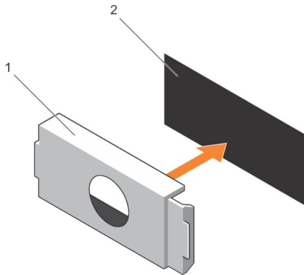
图 44: 卸下和安装电源设备挡片
