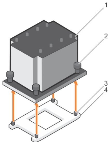
图 21: 卸下和安装处理器
