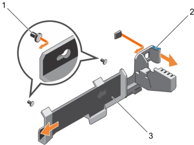
图 29: 卸下和安装电缆固定支架
