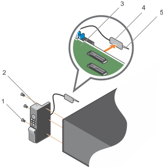
图 58: 卸下和安装控制面板
