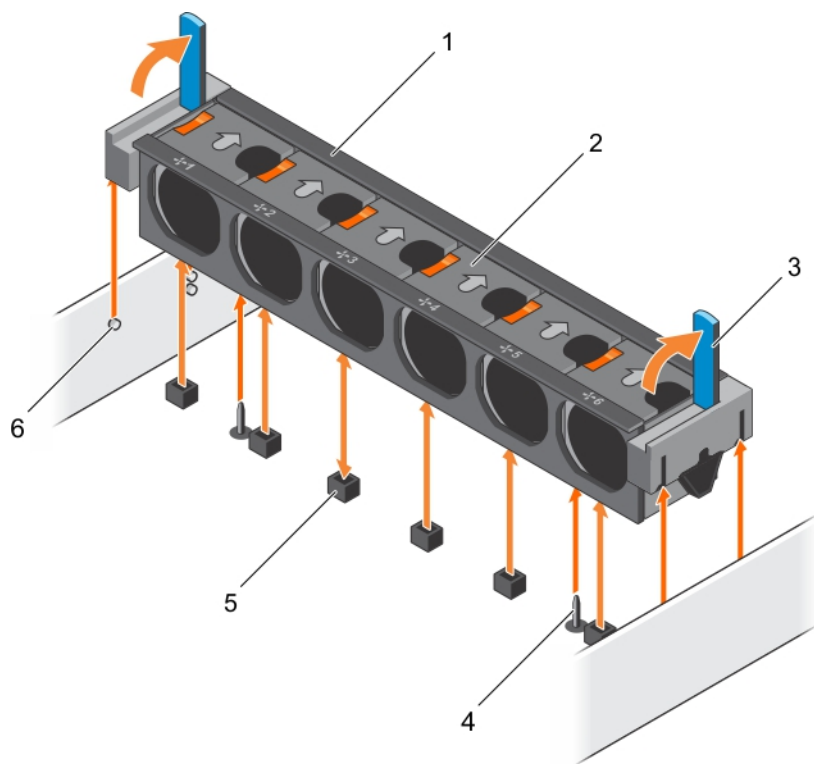
图 15: 卸下和安装冷却风扇部件
