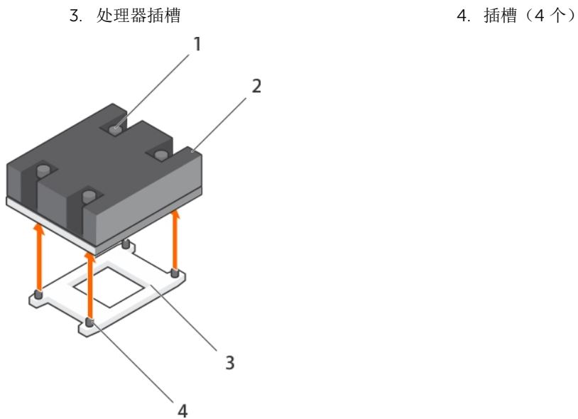
图 23: 卸下和安装处理器散热器
