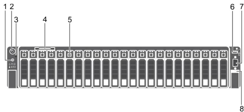
图 1: 2.5 英寸硬盘驱动器或 SSD 机箱
