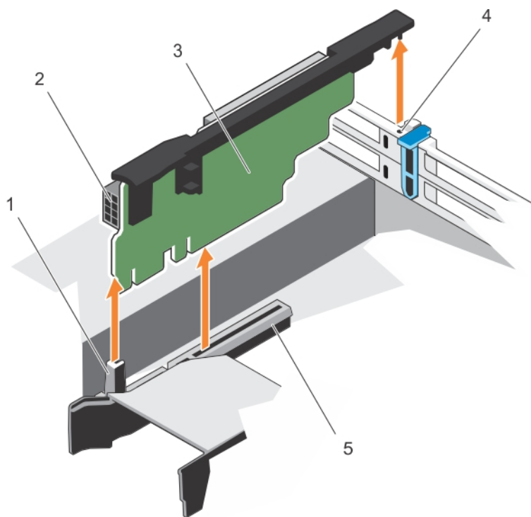
图 37: 卸下和安装扩展卡提升板 3
