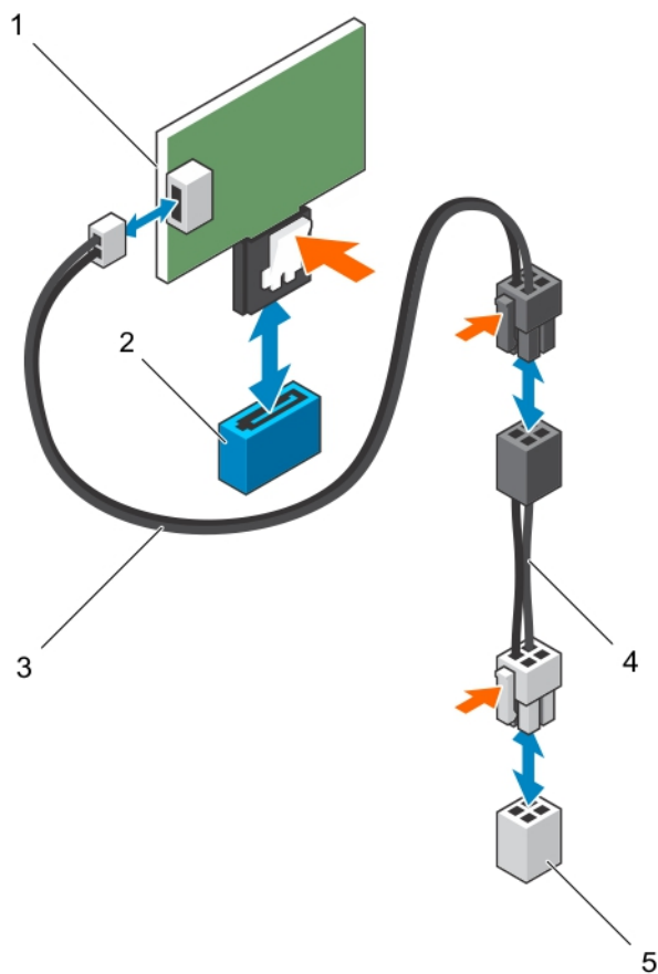
图 20: 卸下和安装 SATADOM
