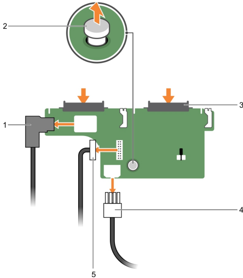
图 57: 卸下和安装可选的 2.5 英寸 (x2) 硬盘驱动器背板
