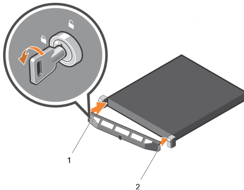
图 10: 卸下和安装前挡板
