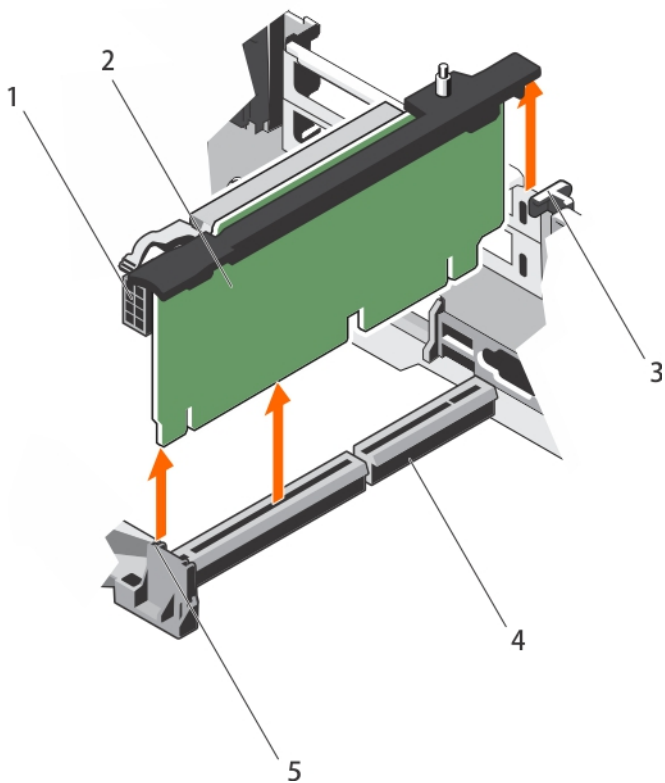
图 35: 卸下和安装扩展卡提升板 2
