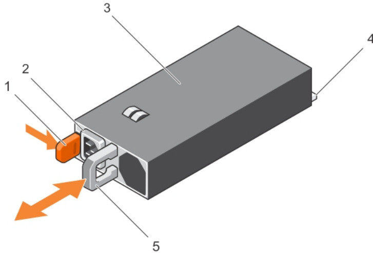
图 45: 卸下和安装交流电源设备
