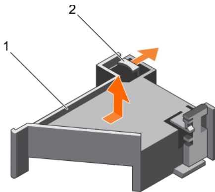
图 27: 卸下和安装 PCIe 卡固定器
