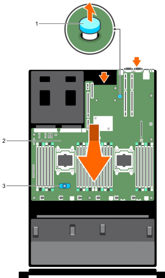
图 47: 卸下和安装系统板
