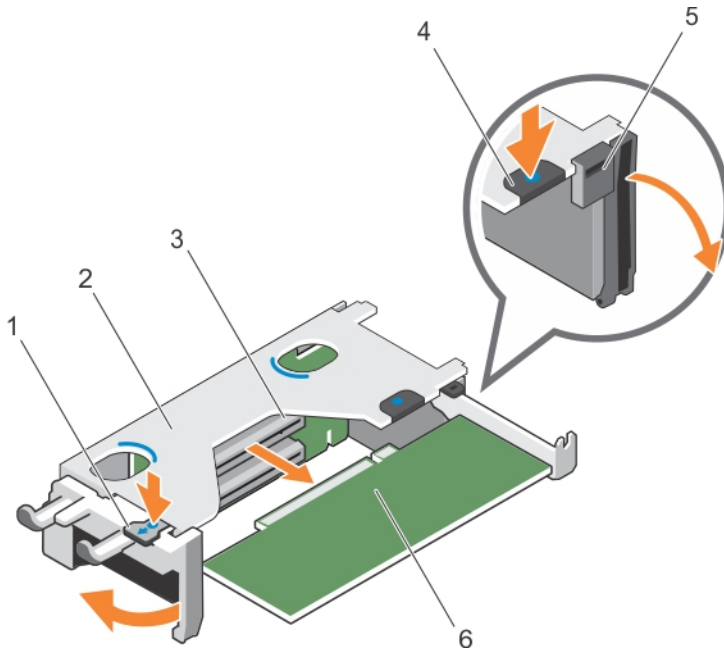
图 32: 在扩展卡提升板 1 中卸下和安装扩展卡
