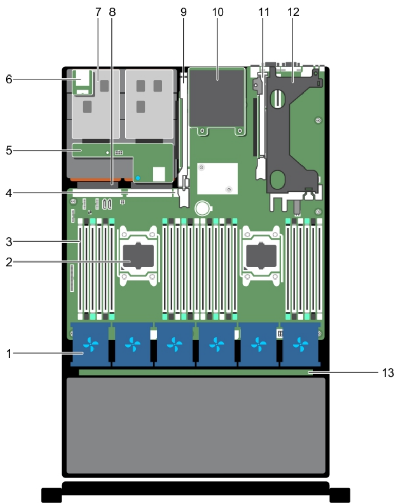
图 12: 系统内部 - Dell XC730xd
