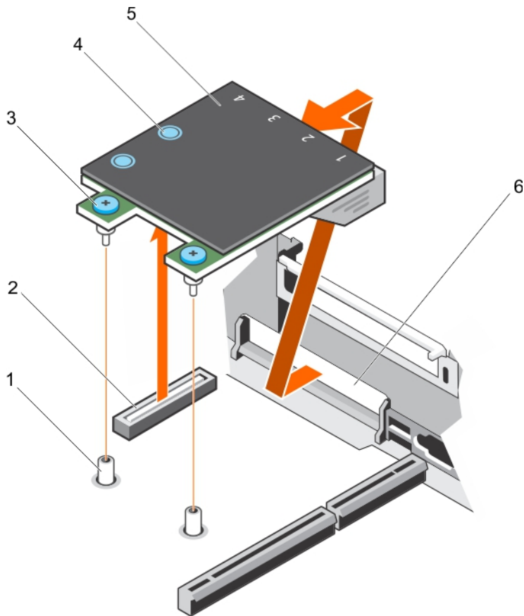
图 41: 卸下和安装网络子卡 (NDC)
