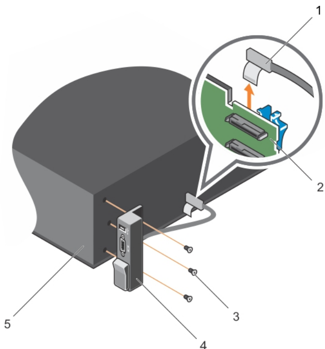
图 59: 卸下和安装 I/O 面板
