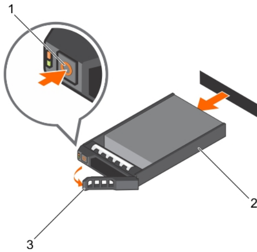
图 52: 卸下和安装热插拔硬盘驱动器
