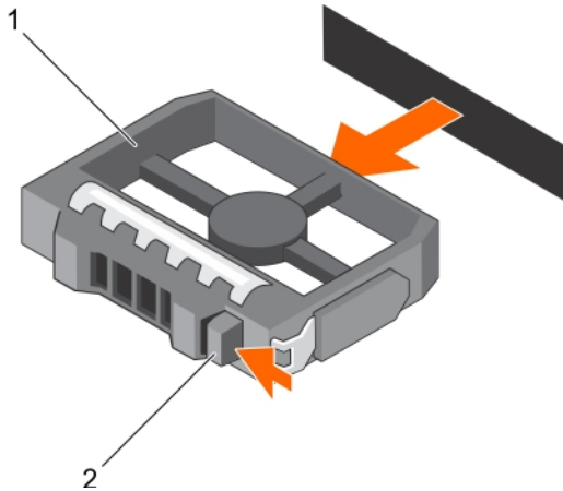
图 51: 卸下和安装 3.5 英寸硬盘驱动器挡片
