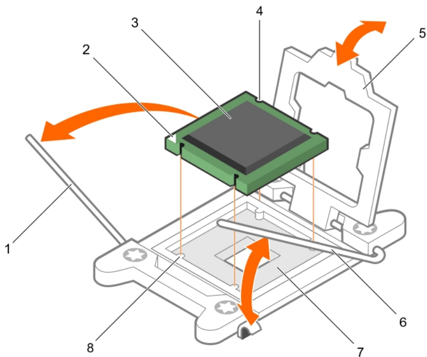
图 25: 卸下和安装处理器
