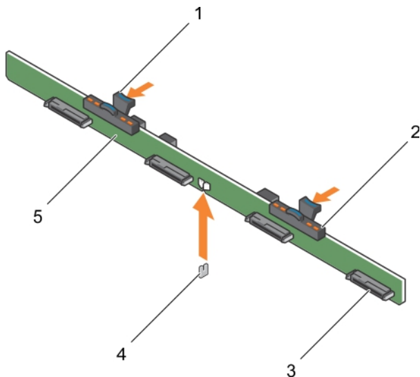
图 60: 卸下和安装 3.5 英寸 (x4) 硬盘驱动器背板
