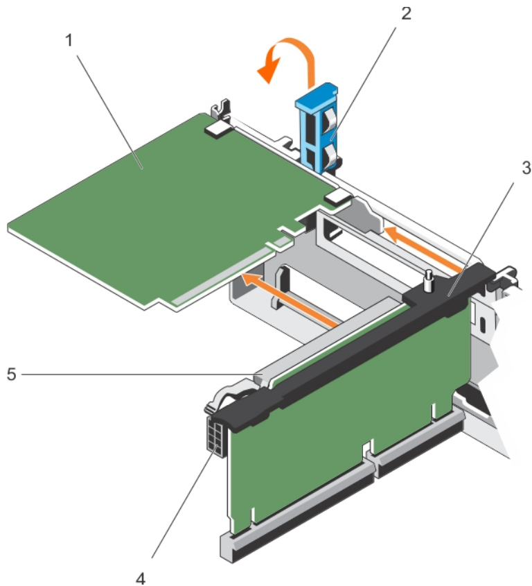
图 31: 在扩展卡提升板 2 或 3 中卸下和安装扩展卡
