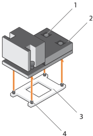
图 22: 卸下和安装处理器散热器
