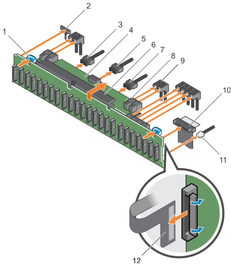
图 54: 卸下和安装 2.5 英寸 (x24) SAS/SATA 背板
