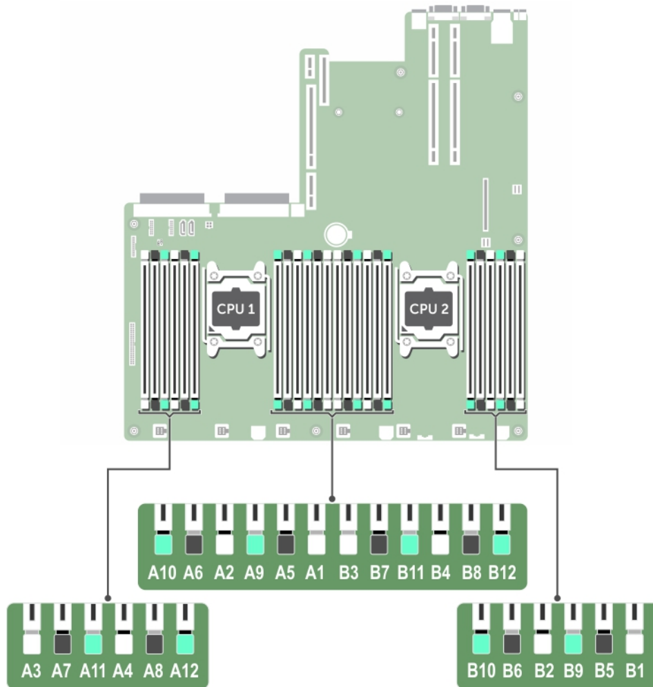
图 16: 内存插槽位置
