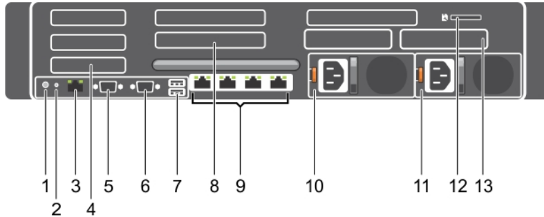
图 6: 背面板功能部件和指示灯
