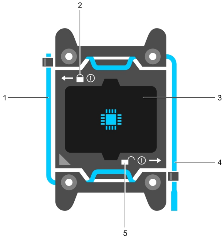
图 24: 处理器护罩
