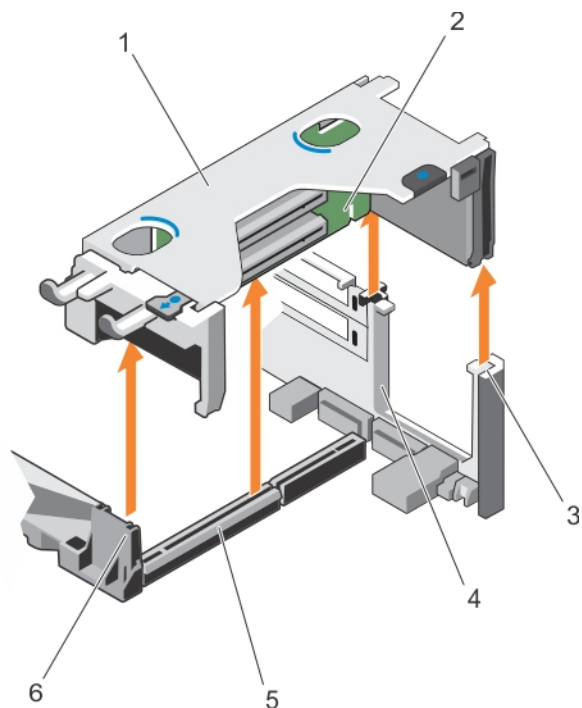
图 33: 卸下和安装扩展卡提升板 1
